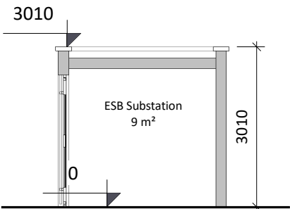
⑦ Section A-A 1 : 100
