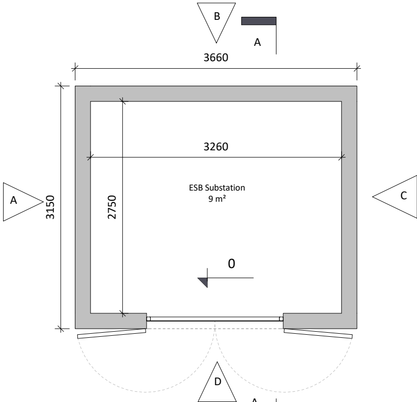
① Floor Plan 1 : 50
