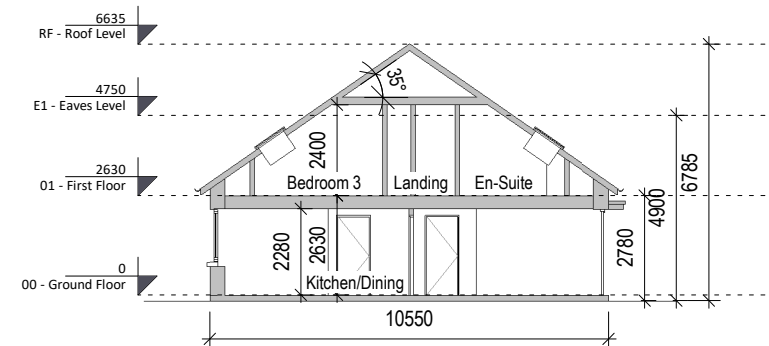
6 Section AA 1 : 200
